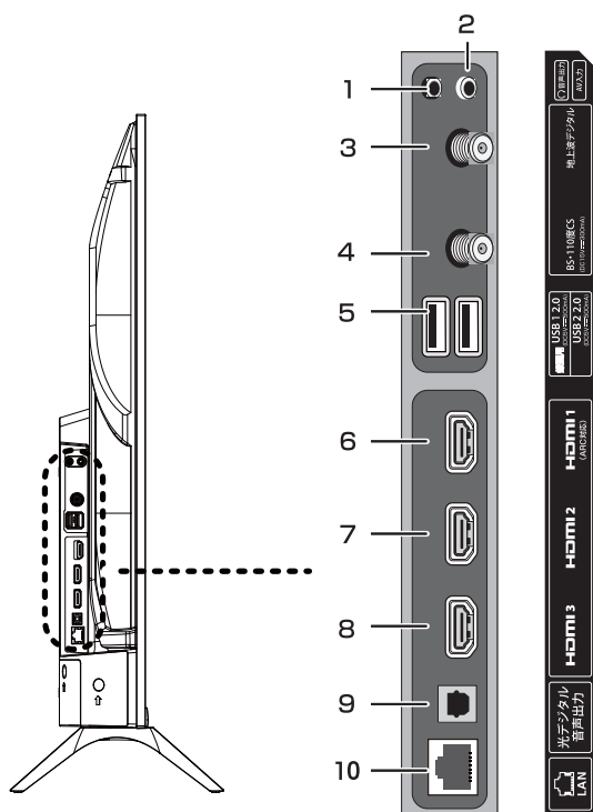
側面 入出力端子部
